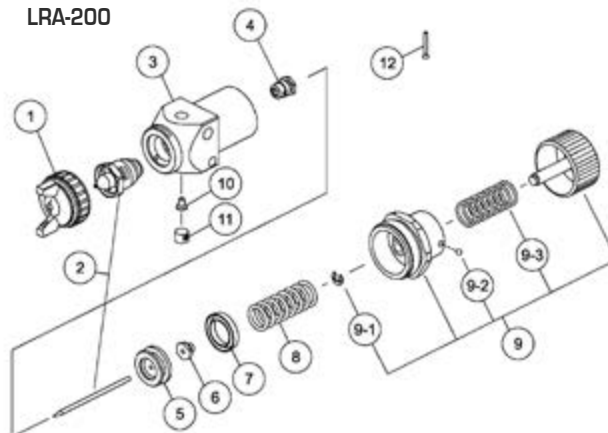
LRA-200
