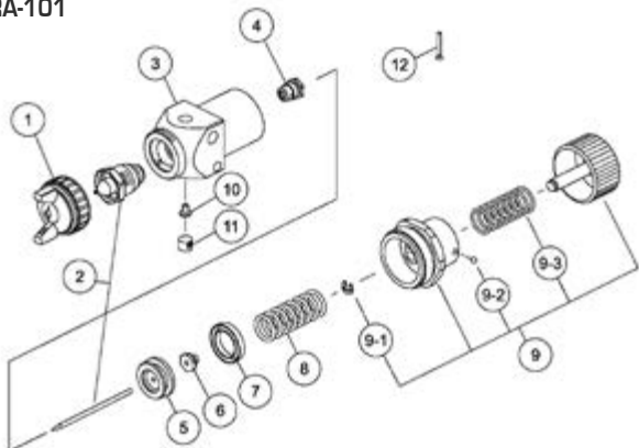
WRA-101
